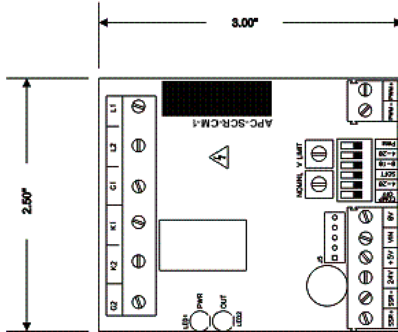
APC-SCR-CM-1 MODULE (ALONE)
